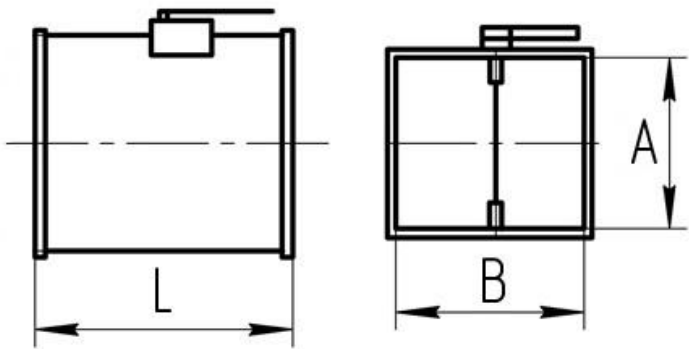
Исполнение с одной лопаткой.
